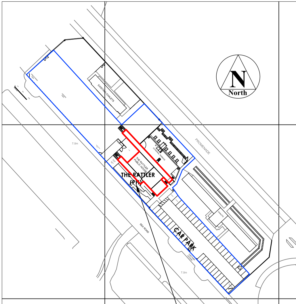
SITE LAYOUT SCALE 1 : 1250
